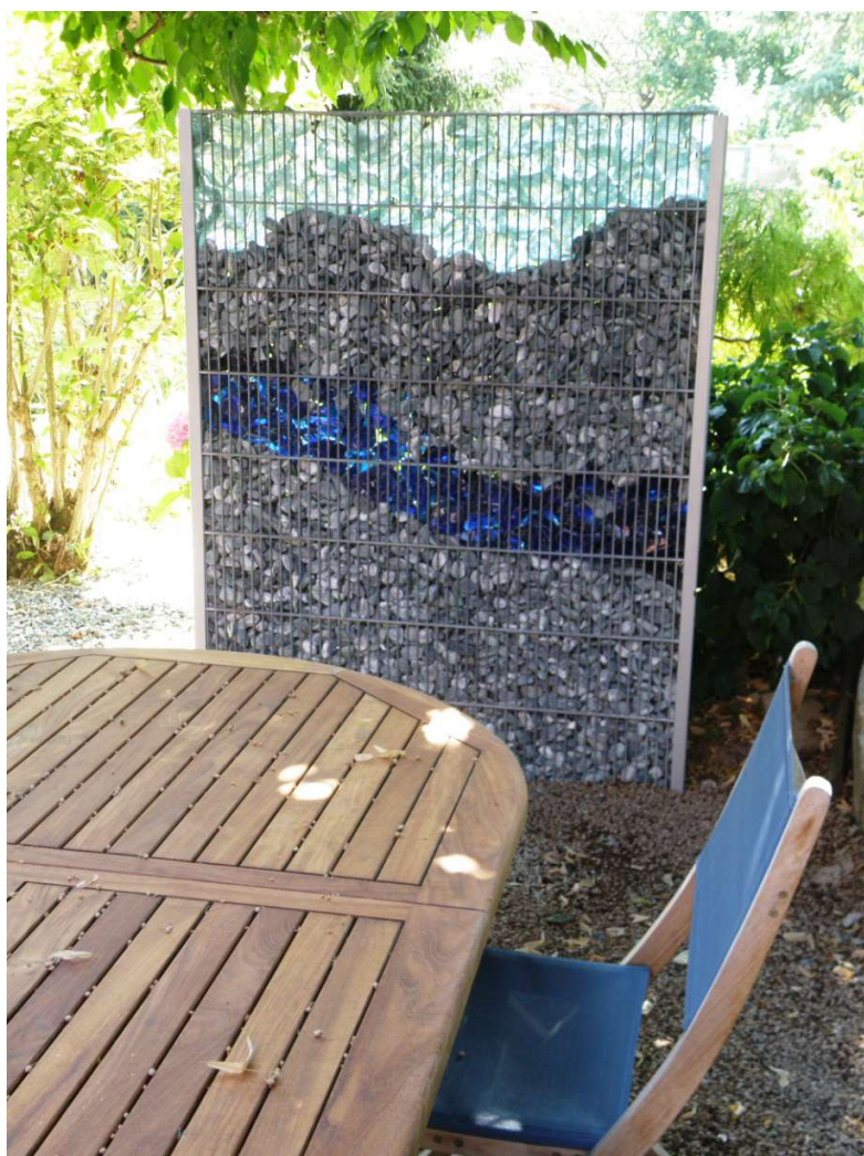
Brise-vue ou brise-vent en gabions en panneaux double fil de 6/5/6, en mailles de 25/200 mm
